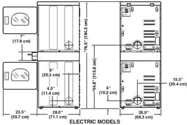
電気式乾燥機 (SSEX-07)
