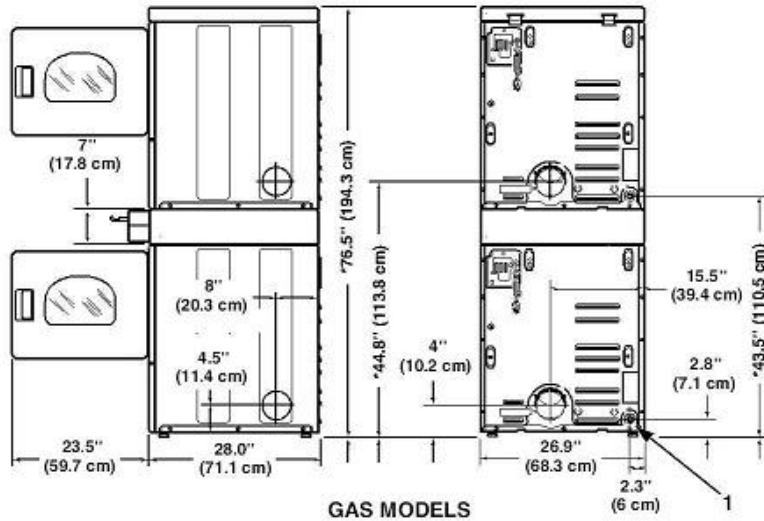
ガス式乾燥機 (SSGX-19)
